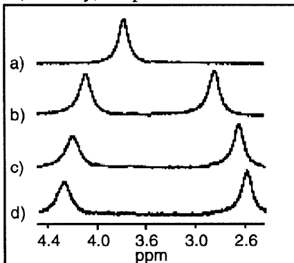
Figure 4 : ^2D -NMR ( CHCl_3 ) : free 3 (a), Na^+ (b), K^+ (c) and Cs^+ (d) complexes
